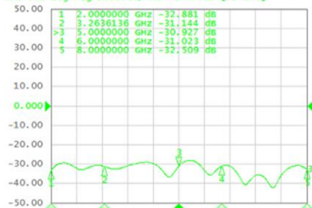
3.隔离度 Isolation
